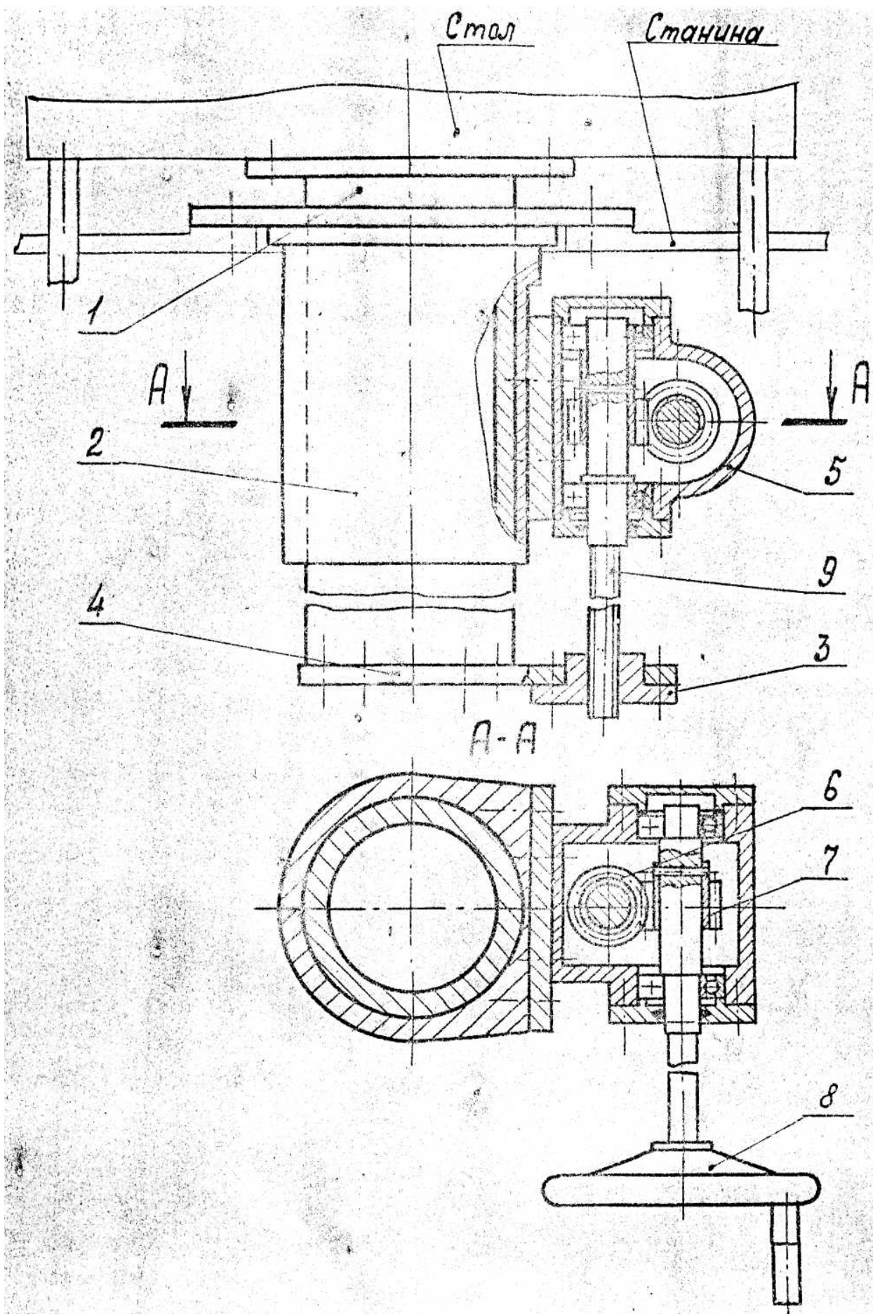
Рисунок 5-Механизм перемещения стола
