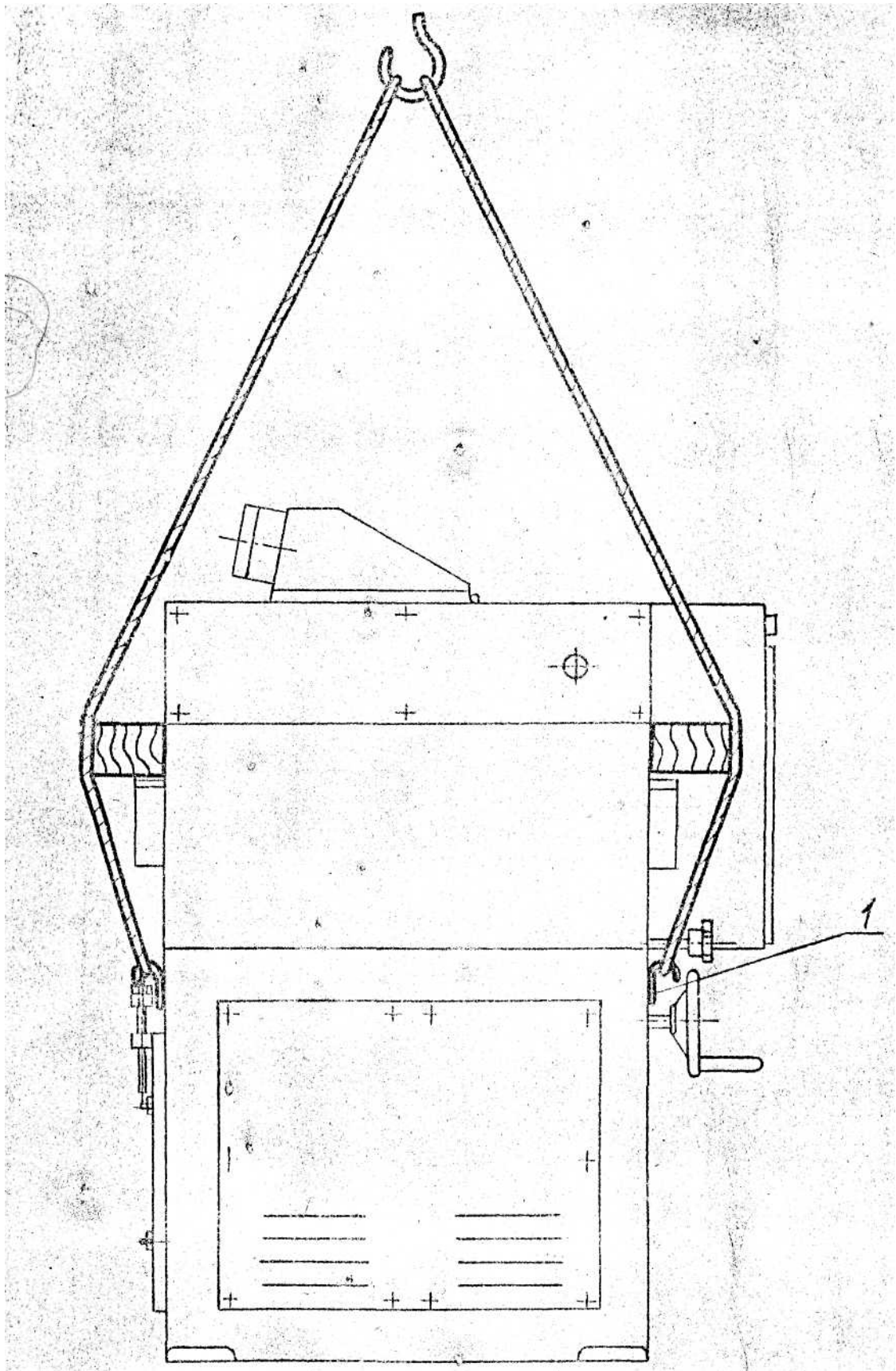
Рисунок 14 - Схема транспортировки станка.
