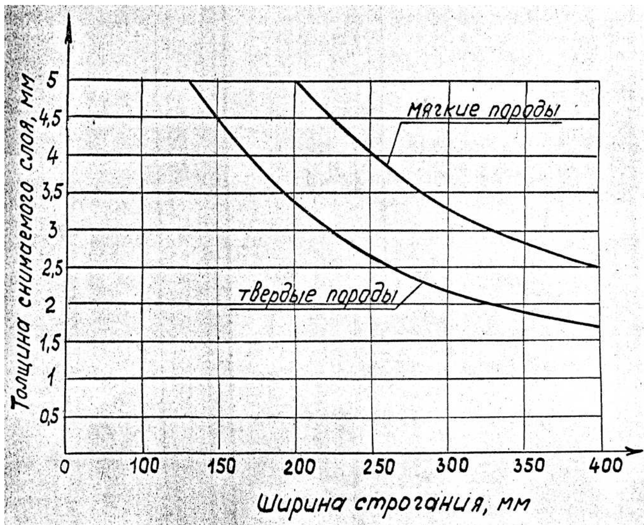
Рисунок 16 - Номограмма
