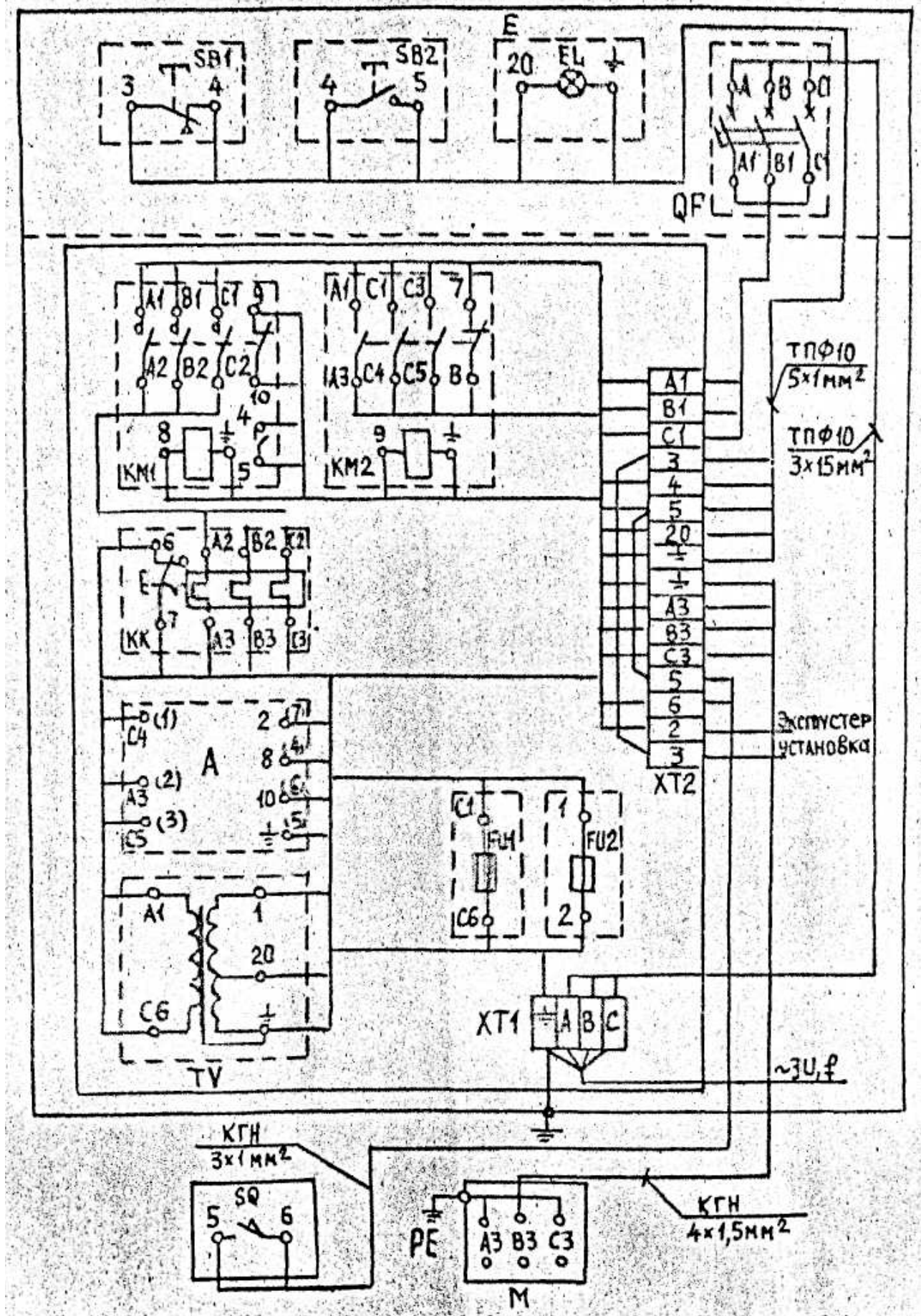
Рисунок 13 – Схема электрическая соединений.
